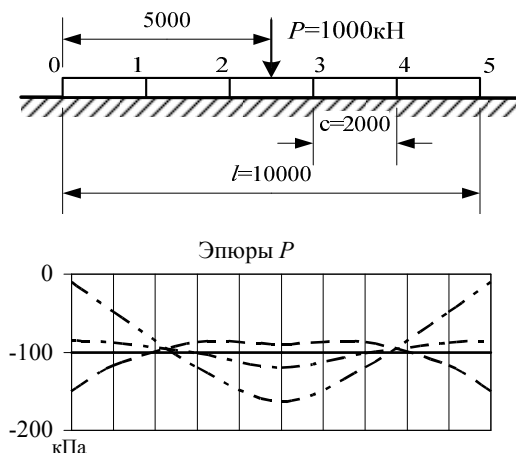
Рис. 3. Эпюры реактивных давлений при c/H = 1/2
